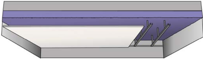
Figure 8 : Plafond suspendu constitué de fourrures et de dispositifs de suspension au support
