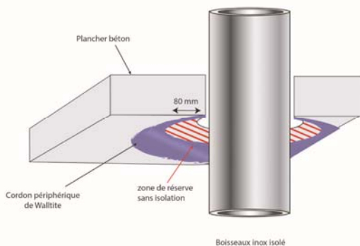
Figure 5 : Isolation autour de conduit de cheminée inox
