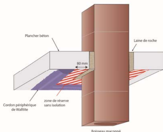
Figure 4 : Isolation autour de conduit de cheminée maçonné
