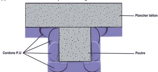
Figure 6 : Cordon d'étanchéité
