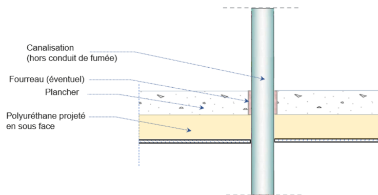
Figure 4 : Traitement d'une canalisation verticale
