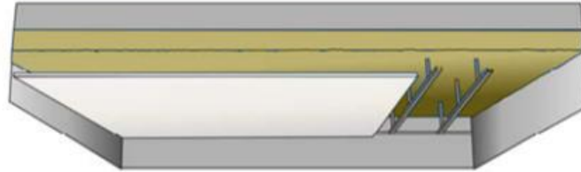
Figure 8 : Plafond suspendu constitué de fourrures et de dispositifs de suspension au support (Avec lame d'air devant l'isolant)
